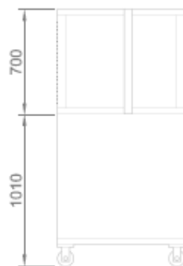
VISTA POSTERIORE + SUPPORTO BACK VIEW + STAND
