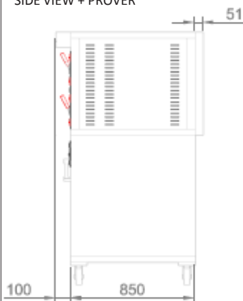
VISTA LATERALE + CELLA DI LIEVITAZIONE SIDE VIEW + PROVER
