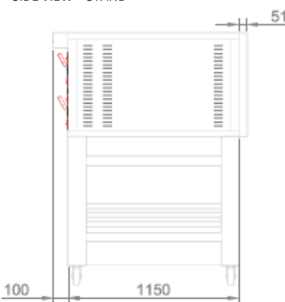
VISTA LATERALE + SUPPORTO SIDE VIEW + STAND
